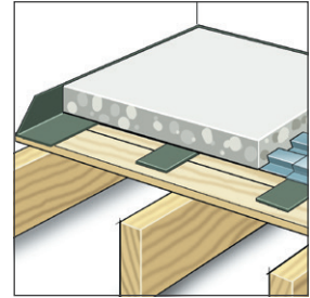
Geluidsislerend op vloerdelen
