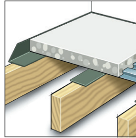
Geluidsislerend op balklaag
