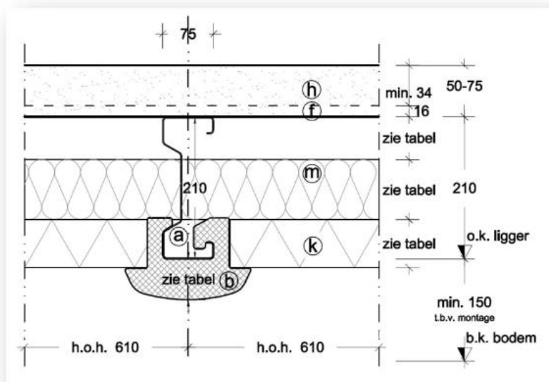
Principe detail: h.o.h. 610 mm
