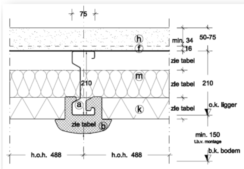
Principe detail: h.o.h. 488 mm
