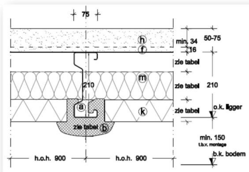
Principe detail: h.o.h. 900 mm
