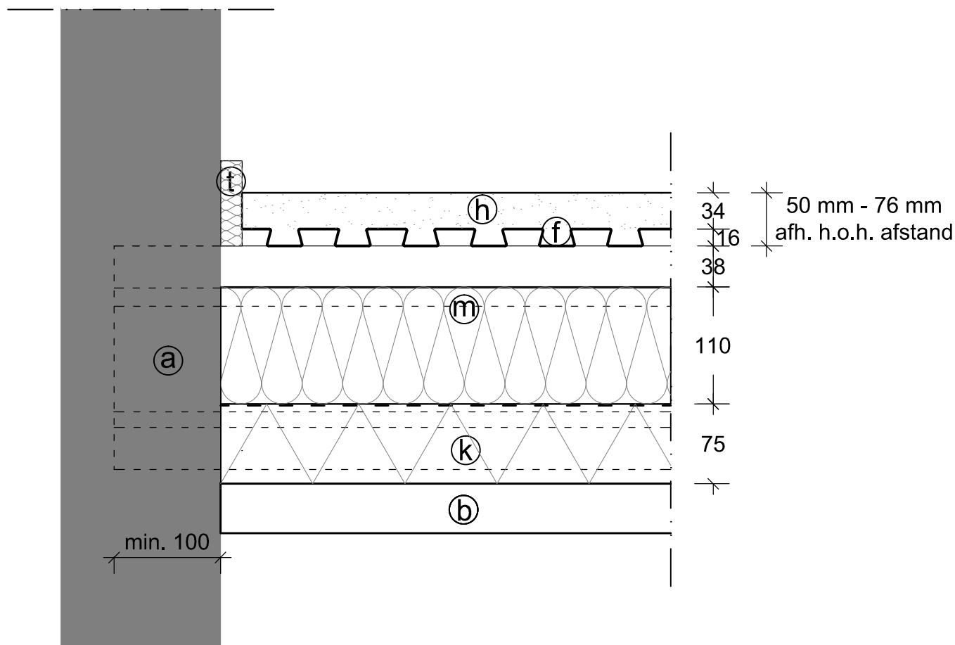
Detail oplegging in bestaande bouwmuur
