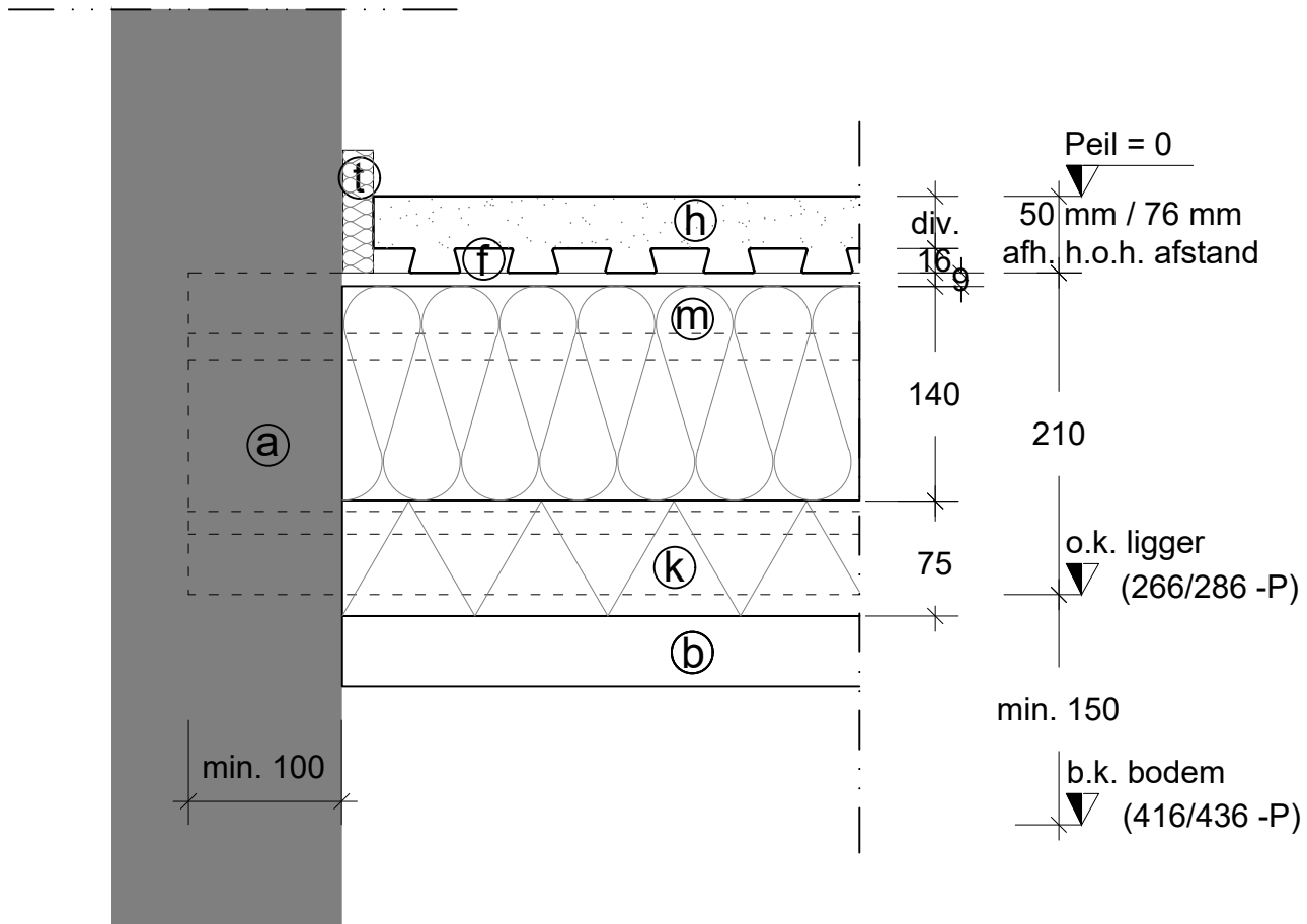
Detail oplegging in (bestaande) bouwmuur
