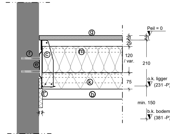
Detail muurprofiel
