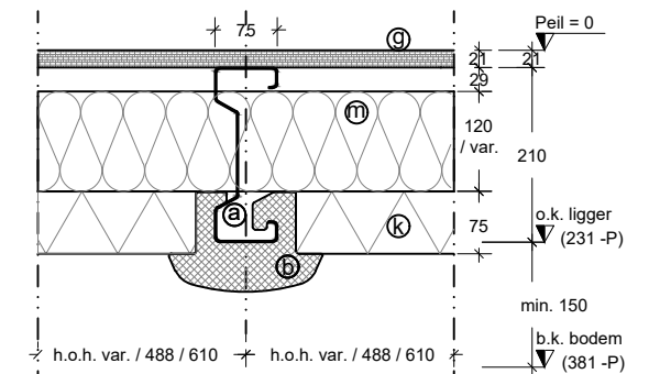
Detail profiel
