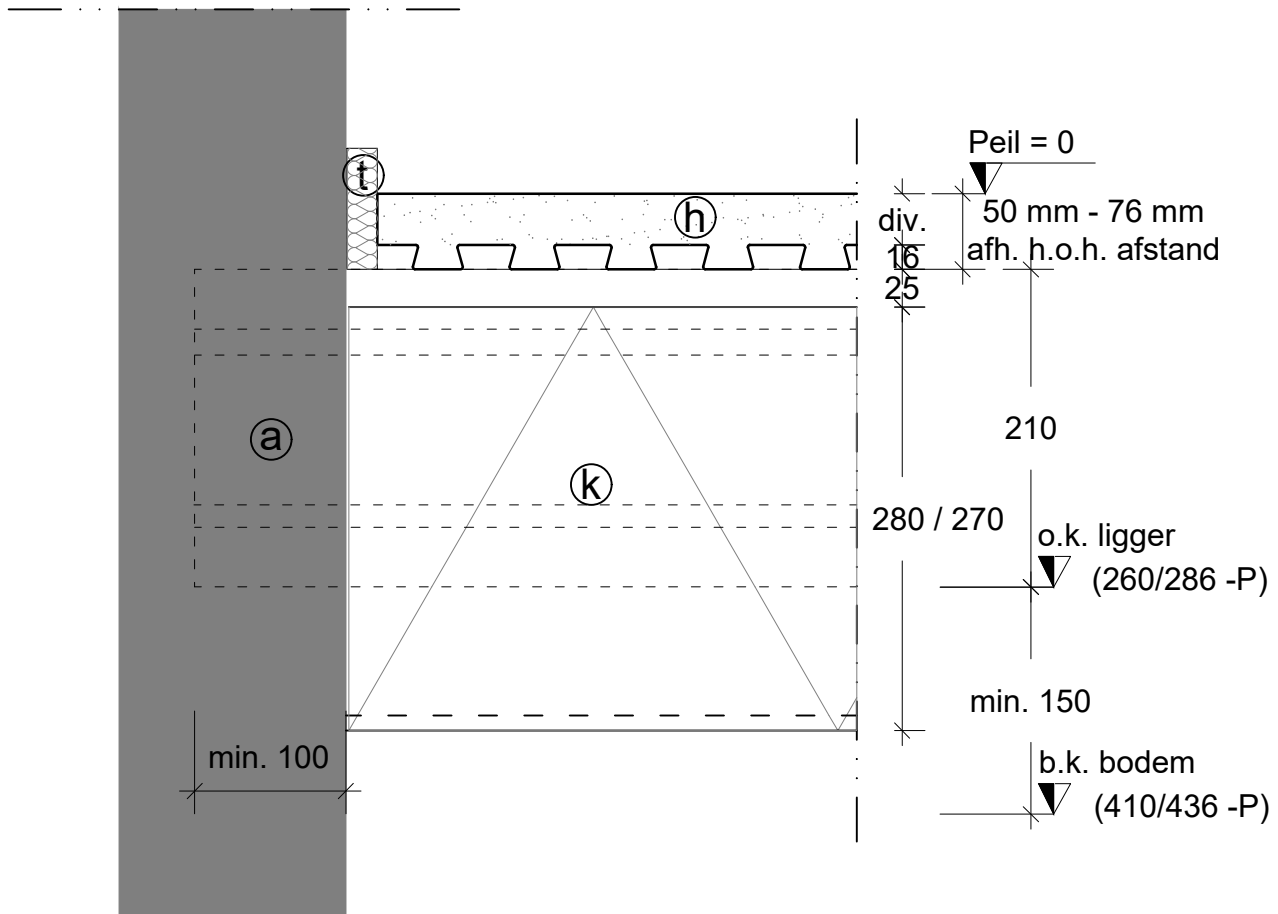
Detail oplegging in (bestaende) bouwmuur
