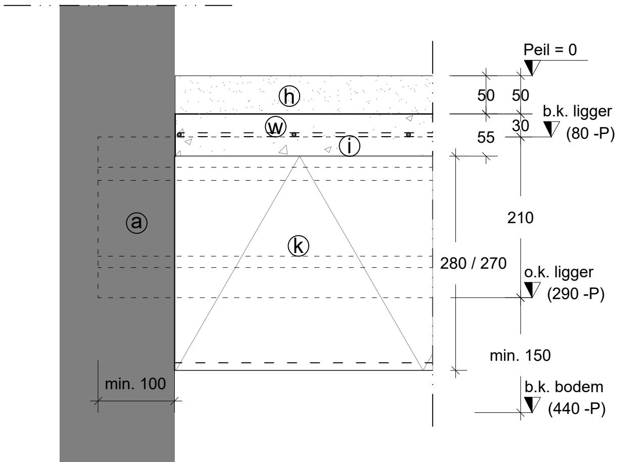
Detail oplegging in (bestaende) bouwmuur
