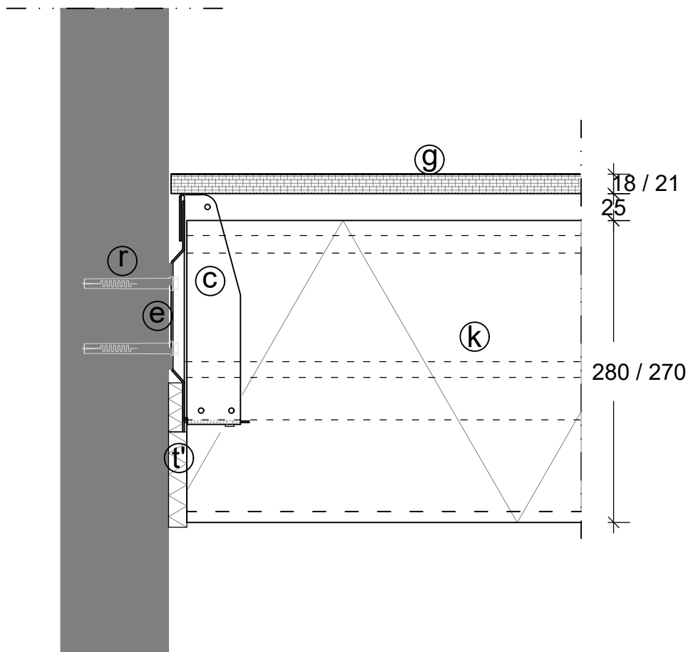
Detail muurprofiel
