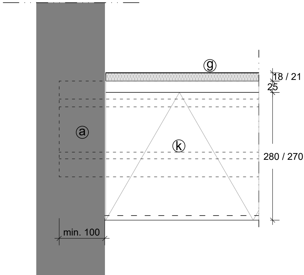
Detail oplegging in (bestaande) bouwmuur
