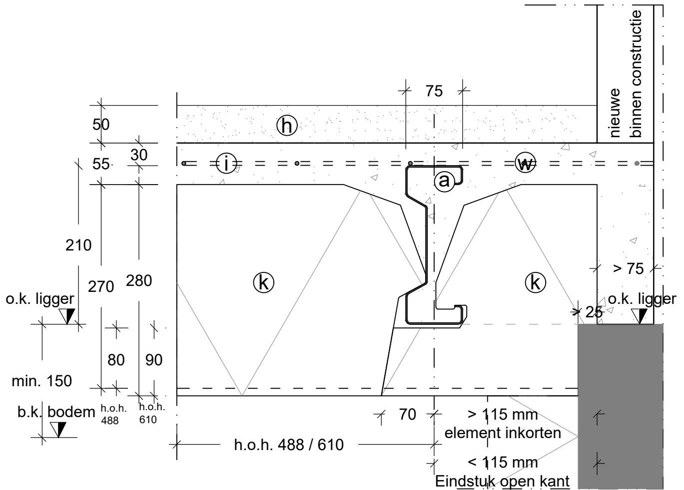
Detail 2 oplegging vulelement - Nieuwbouw
