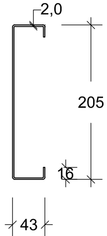
Doorsnede
